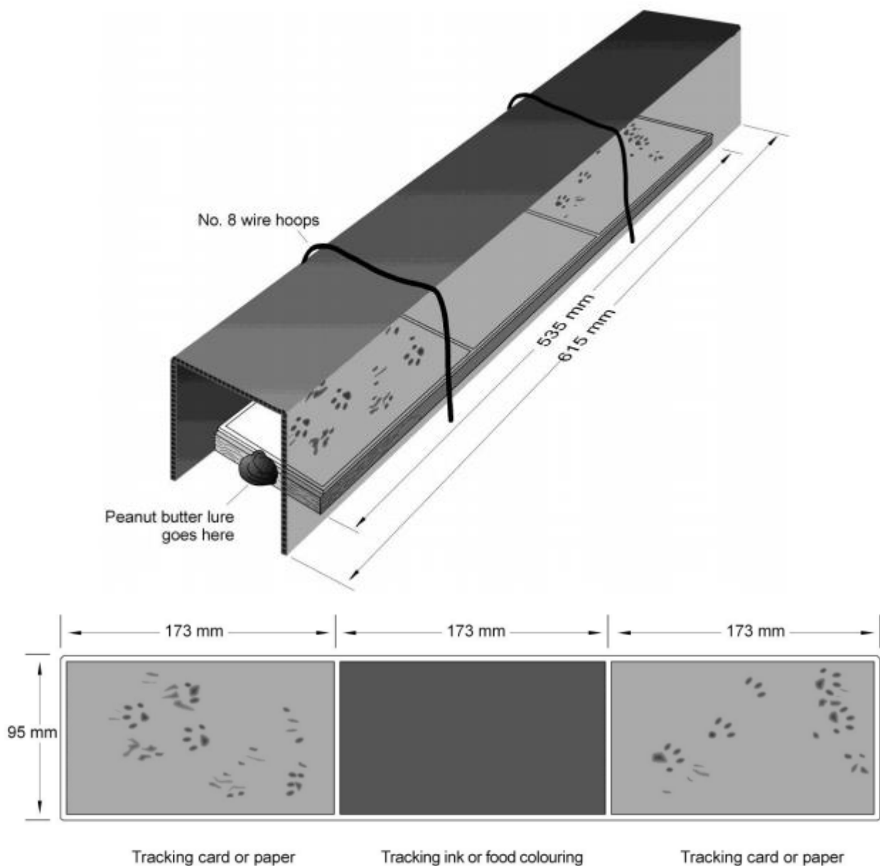
Figuur 7. Schematische weergave van een sporentunnel (Gillies & Williams, 2013). In het centrale deel bevindt zich een inktpad en aan weerszijden papier waarop de pootafdrukken vervolgens zichtbaar worden (zie voorbeeld onder de tunnel). De beoogde soort kan eventueel worden gelokt door visolie of iets dergelijks bij de ingang van de tunnel te leggen.
