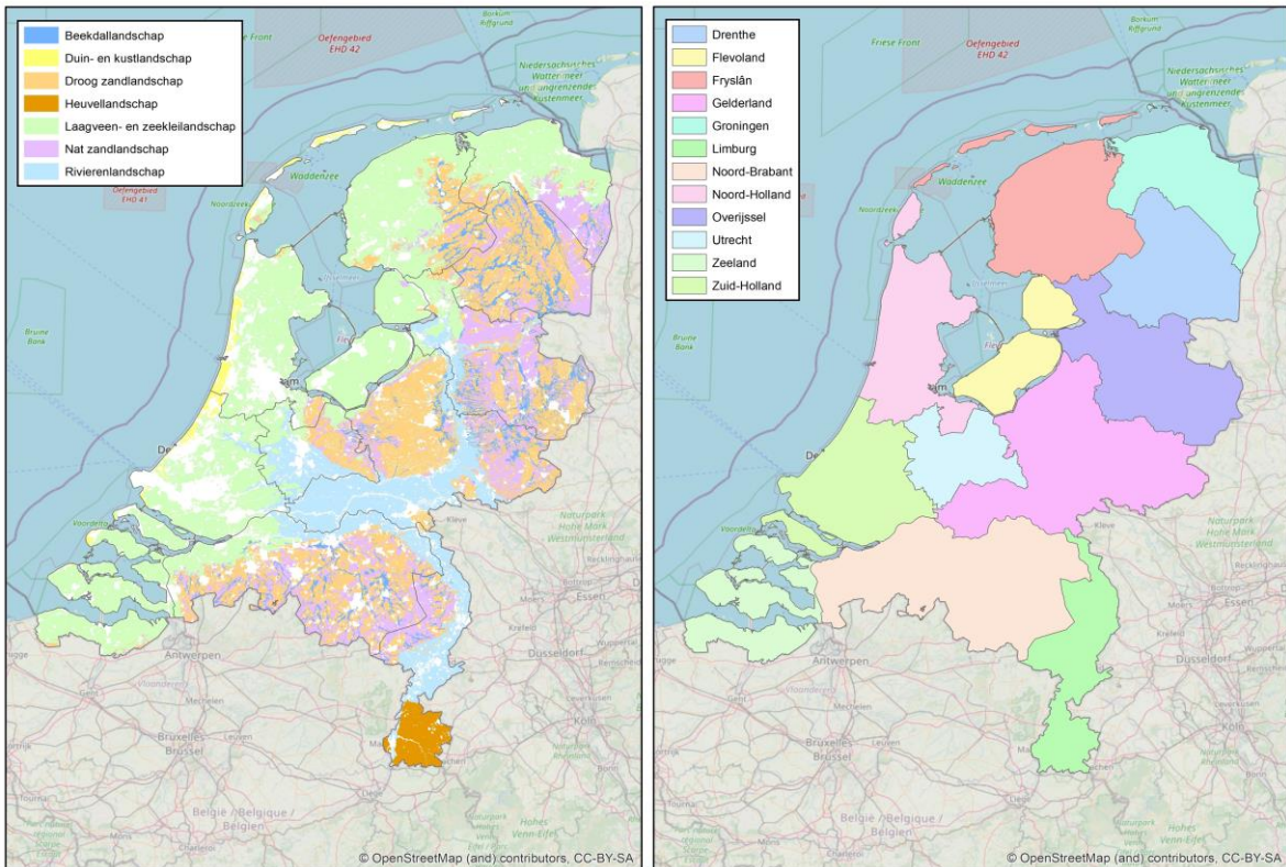
Figuur 2: De indeling van landschappen (links) en regio's (rechts) als hoogste schaalniveau voor Basiskwaliteit Natuur. De landschapsindeling volgt die van het Kennisnetwerk Ontwikkeling en Beheer Natuurkwaliteit (OBN). De landschapstypen 'grote zoete wateren', 'zee en wad' en 'cultuurlandschap' worden op deze kaart niet weergegeven. De kaart is samengesteld op basis van de Landschapsleutel. Niet-gekleurde (witte) vlakken omvatten de stedelijke gebieden. De regionale indeling volgt de provinciale grenzen.
